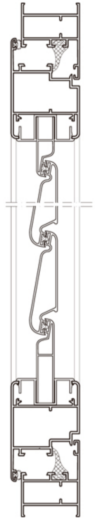
Sección característica
